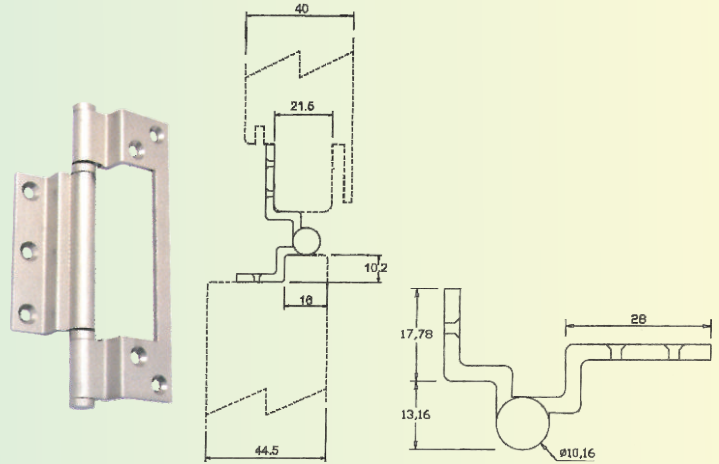
125 SEWING HINGE
